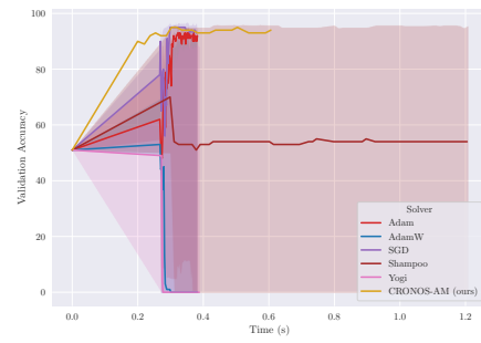
(b) ImageNet-171
