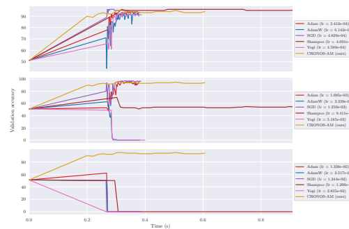
(b) ImageNet-171
