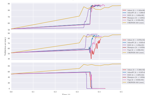
(d) ImageNet
