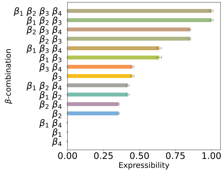
(b) s_L
