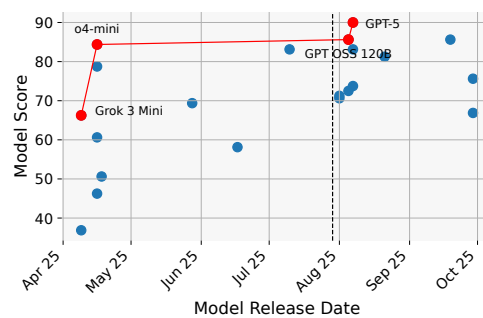
(d) Time-Pareto frontier for CMIMC
