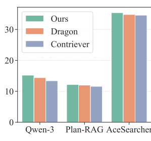
(a) MusiQue
