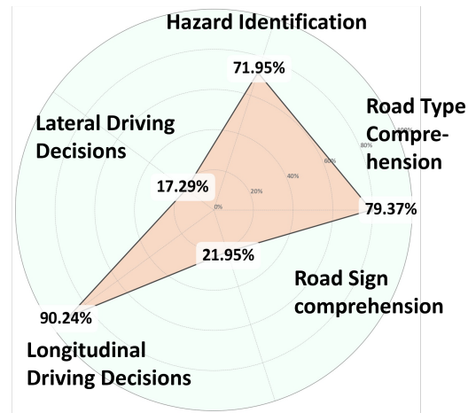
(d) Qwen-Turbo
