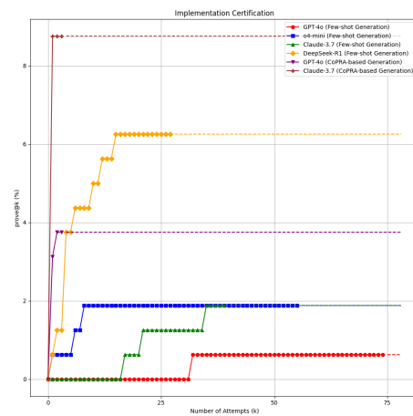
(d) Implementation Certification (prove@k)
