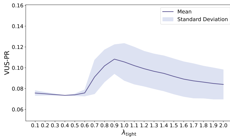
(b) \lambda_{tight}
