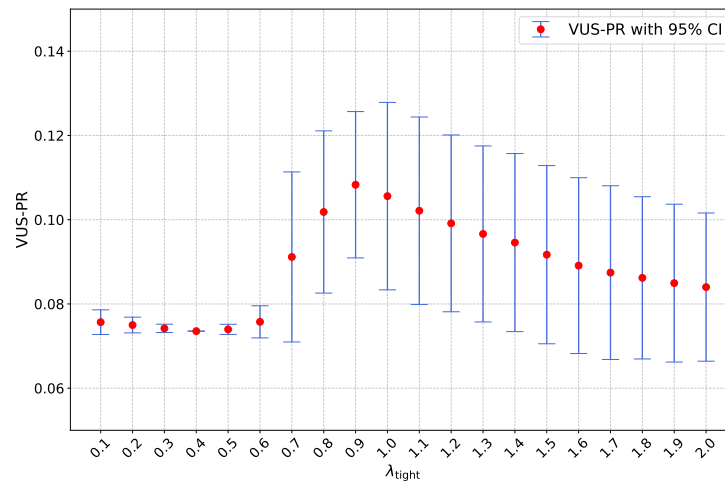
(b) \lambda_{tight}
